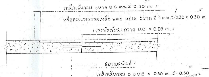
แบบขยาย CONTRACTION JOINT
