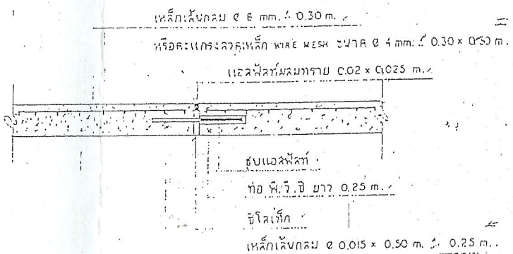
แบบขยาย EXPANSION JOINT
