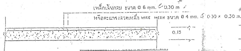
ขยายการเสริมเหล็กถนน คสล.
